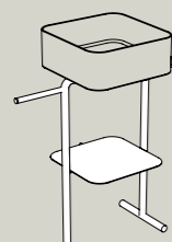
STRUTTURA/RIPIANO FRAME/SHELF S7810007/R78100 43x30xh75 cm
