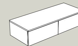
CASSETTO DOPPIO DOUBLE DRAWER MSC115 120x47,7xh25 cm
