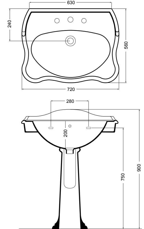
06040 colonna_pedestal
