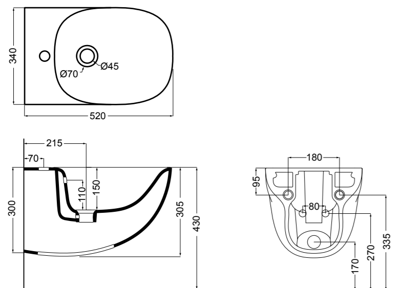
30020 bidet sospeso_wall hung bidet
