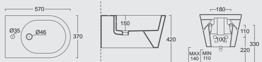
Bidet sospeso Hide Round Hide Round wall hung bidet
