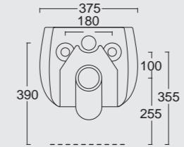
Cod. 33120101 Vaso sospeso Nur Nur WC wall hung
