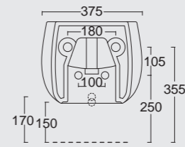
Cod. 33130101 Bidet sospeso Nur Nur bidet wall hung
